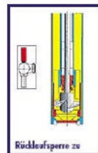
Funktionsschema: Pumpe F 425 Rücklaufsperre zu
