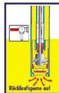
Funktionsschema: Pumpe F 425 Rücklaufsperre auf
