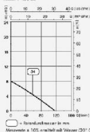
Motor F 460 Ex
